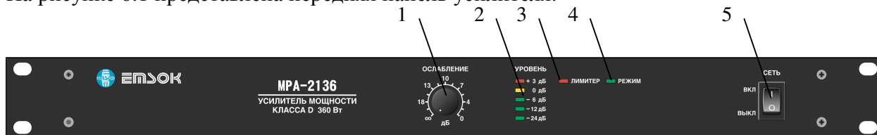
Рисунок 6.1. Передняя панель усилителя. 1 – Регулятор громкости, 2 – индикатор уровня, 3 – индикатор перегрузки, 4 – индикатор режима работы, 5 – выключатель питания.
